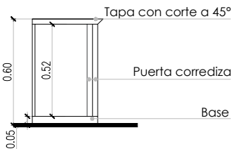
CORTE - IV. MUEBLE DE GUARDADO LAQUEADO
