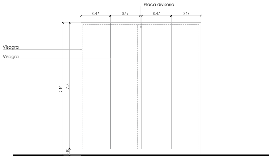
VISTA - V. PLACARD DE GUARDADO LAQUEADO
