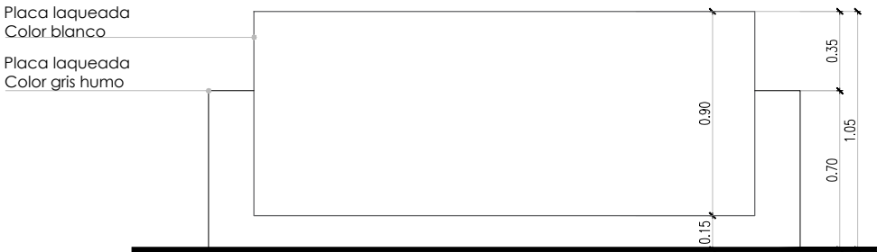
VISTA FRENTE - I . PUESTO SIMPLE
