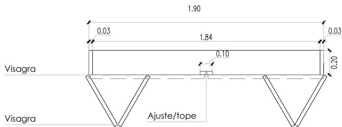
PLANTA - V. PLACARD DE GUARDADO LAQUEADO
