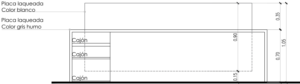
VISTA TRASERA - I . PUESTO SIMPLE
