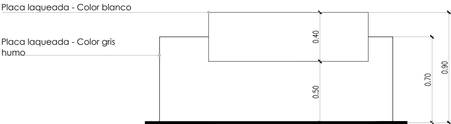
VISTA FRENTE - II. PUESTO SIMPLE
