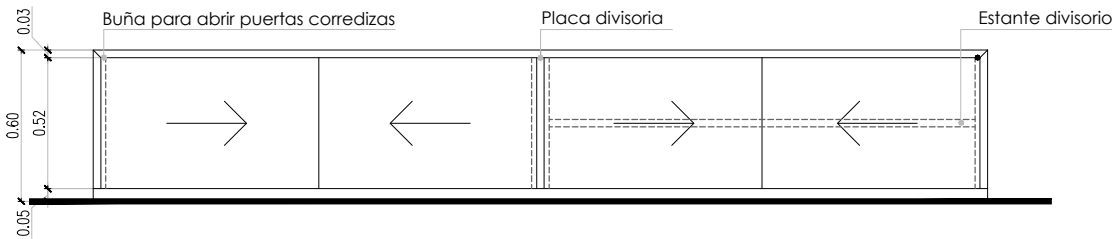
VISTA - IV. MUEBLE DE GUARDADO LAQUEADO
